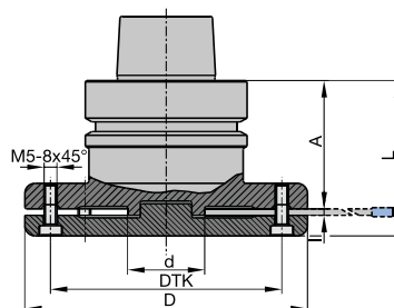
Rychloupínací montážní přípravek pro kleštinové upínače HSK63F a ISO30 při výměně nástroje
