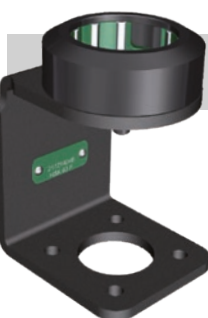
Rychloupínací montážní přípravek pro kleštinové upínače HSK63F a ISO30 při výměně nástroje
